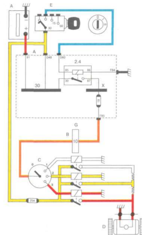
Электросхема питания вентилятора системы вентиляции и отопления салона в автомобилях до модели 1983 г. с радиальным вентилятором
